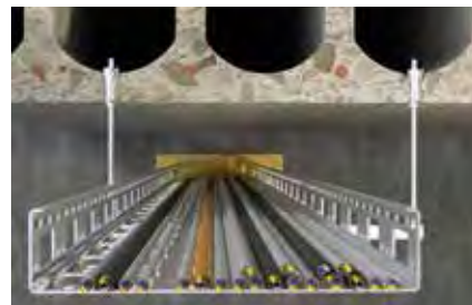
Nosné systémy káblov montované k dutinovým panelom z predpätého betónu
